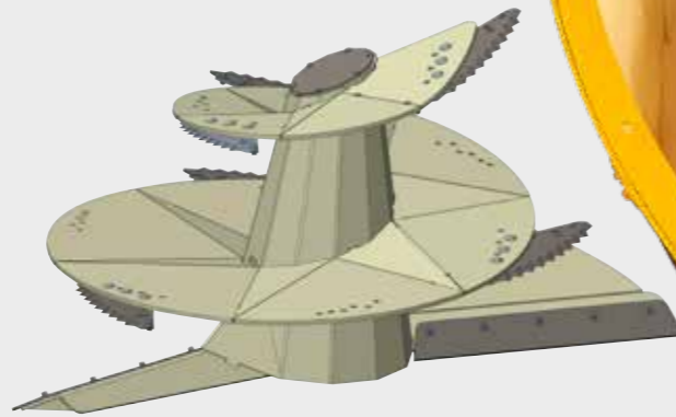
Шнек "Mélange" с обычным шагом, оснащён 6 / 8 / 10 оборотными ножами.
