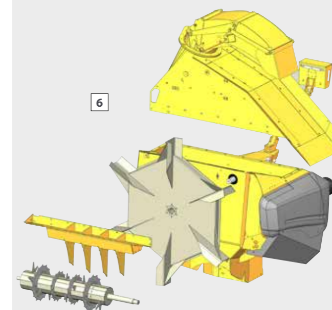
Рисунок 3D блока раздачи кормов и соломы SPIRMIX Jet
