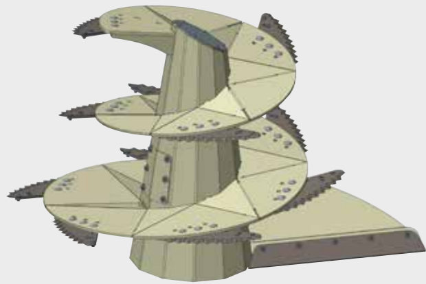
Шнек "Fibre" с обычным шагом, предназначен для измельчения сена, соломы, тюков в плёнке. Оснащён 11 оборотными ножами
